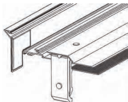
Pormenor do esquadro base e esquadro de alinhamento
