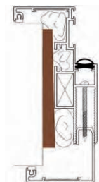
Fixação do perfil base com o perfil de ajuste
